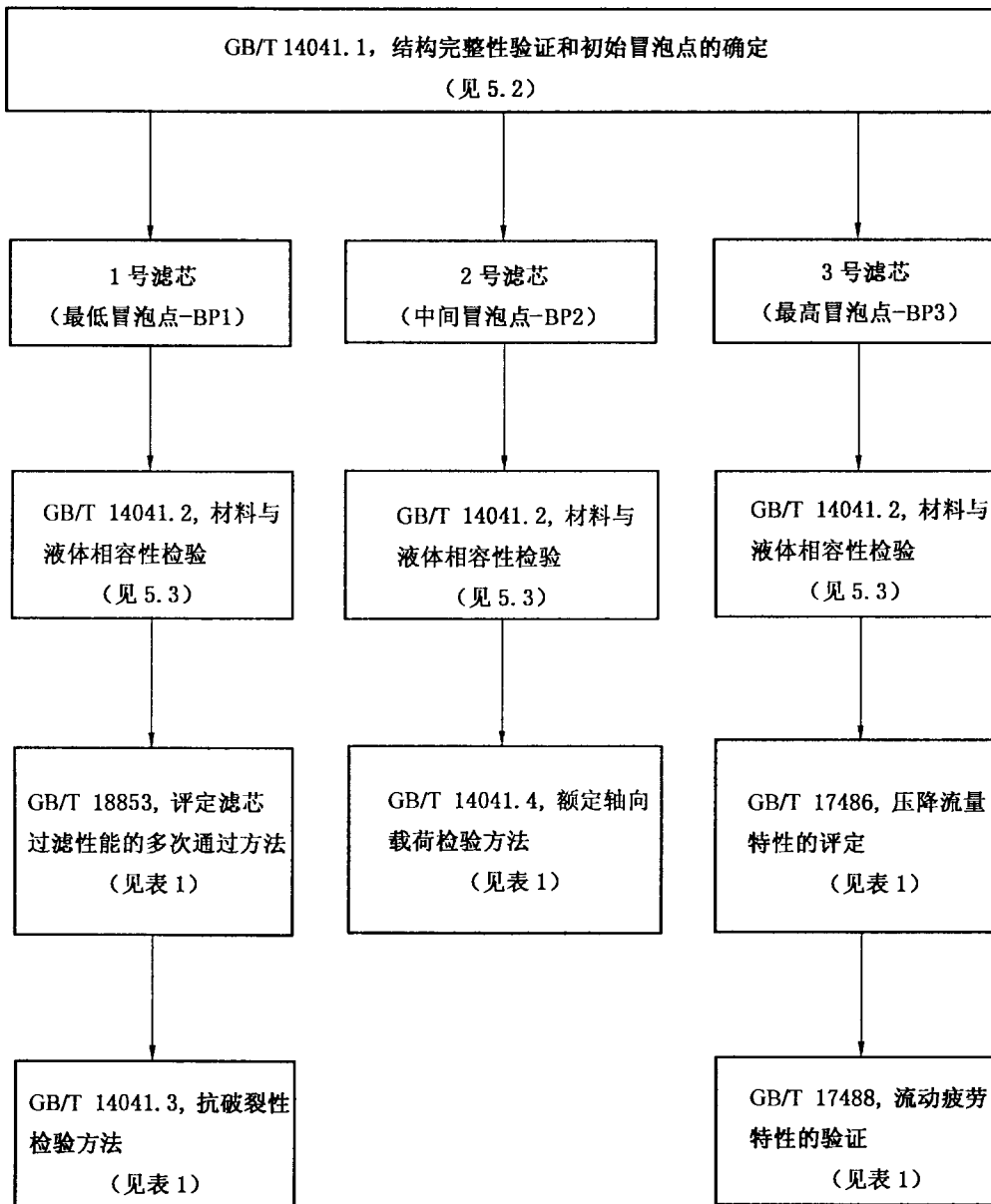
图 1 试验程序
