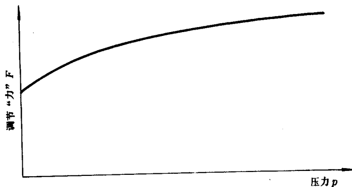
图 4 控制部件调节“力”曲线
