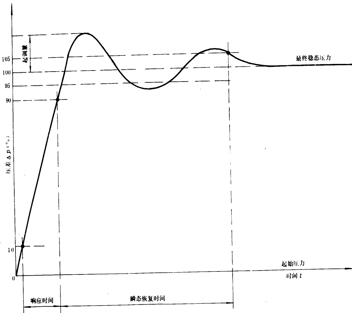
图 4 控制部件调节“力”曲线
